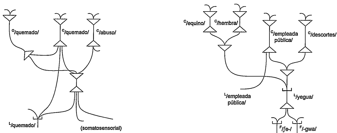
Figura 14. Condensaciones (nodos 'y' + 'y' [ \nabla ]; nodos 'y' + 'o' [ \sqcup ])
